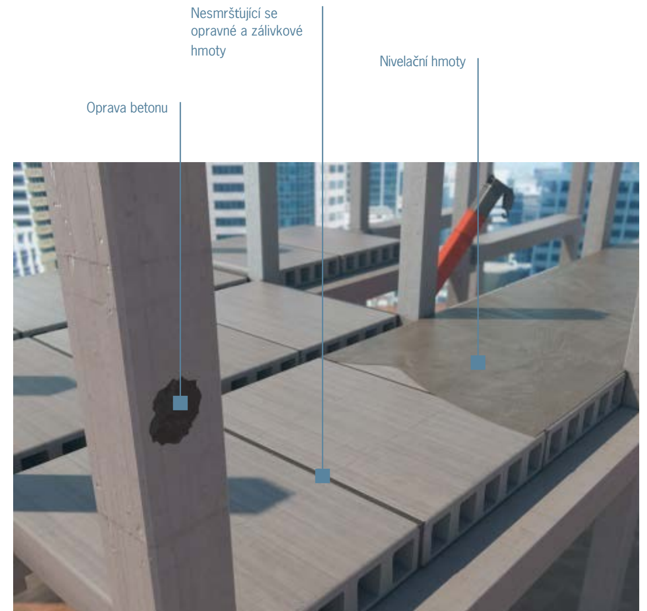
Řešení ARDEX pro prefabrikované prvky
